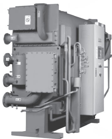
16LJ013 med en kyleffekt på 400Kw.
